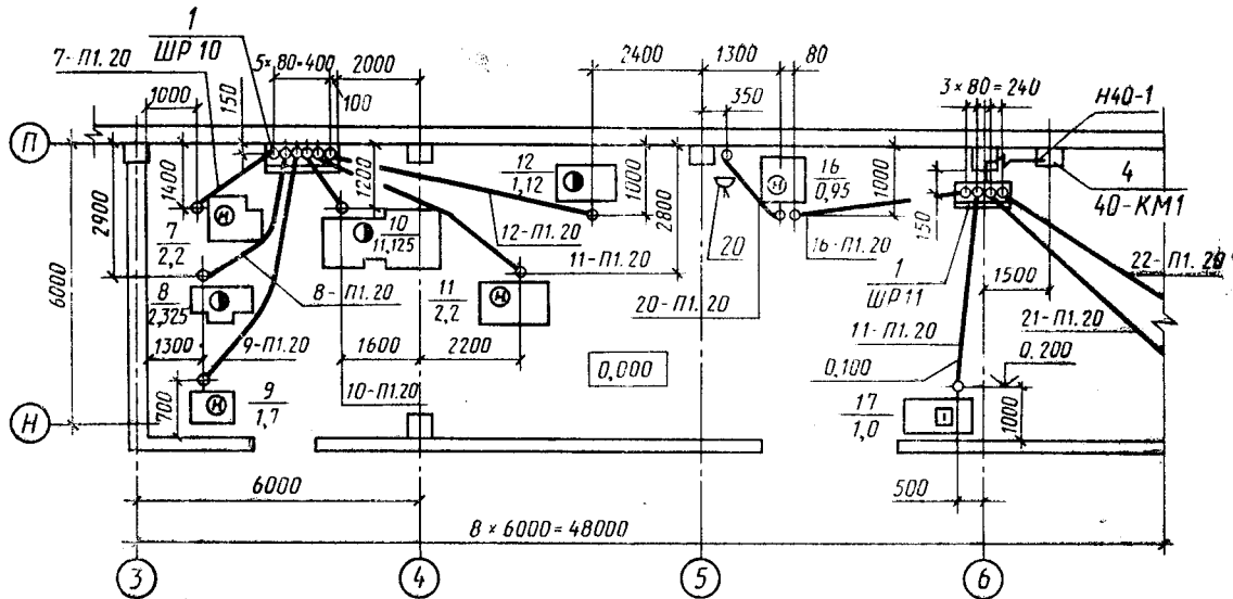
Трубы проложить на отм. — 0.100 и концы их вывести на 200 мм над уровнем чистого пола Черт. 4
